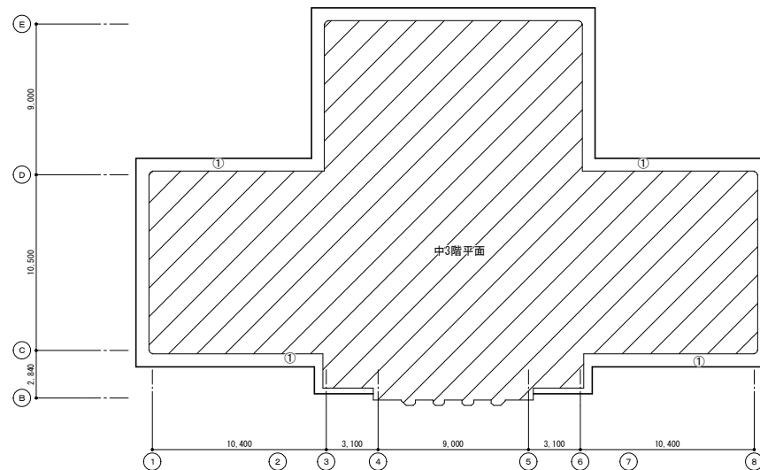
底伏図 S=1/200
